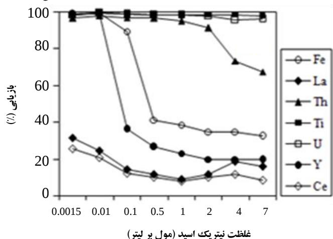
شکل ۱. تغییرات میزان بازیابی یون های فلزی با سیانکس ۲۷۲ رقیق شده در کروژن، به عنوان تابعی از غلظت نیتریک اسید (شرایط: غلظت متوسط یون فلزی: 10^{-4} \text{ mol L}^{-1} ، غلظت سیانکس ۲۷۲: 0.1 \text{ mol L}^{-1} ).
