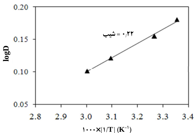
شکل ۵. اثر دما بر استخراج توریم.
