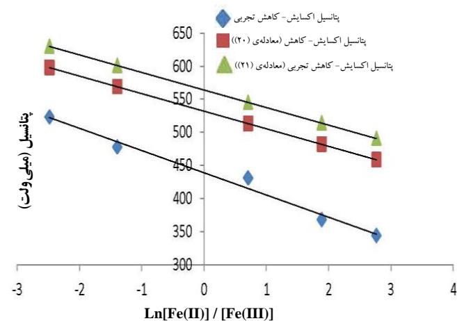
شکل ۶. مقایسه‌ی تغییرات پتانسیل اندازه گیری شده با پتانسیل محاسبه شده از رابطه‌ی نرنست در آزمایش با چگالی پالپ ۱۰٪.
