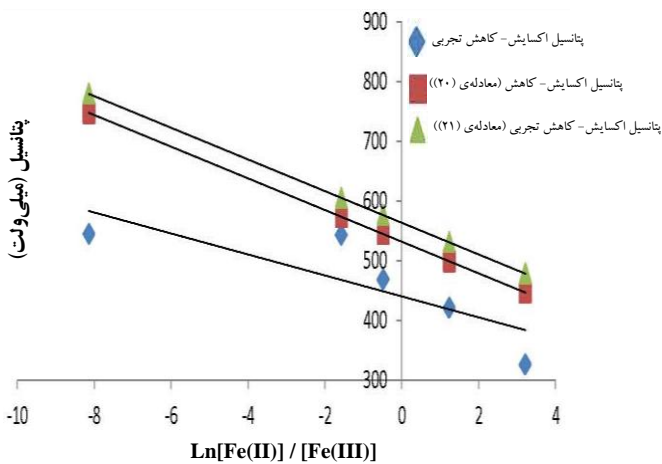
شکل ۵. مقایسه‌ی تغییرات پتانسیل اندازه گیری شده با پتانسیل محاسبه شده از رابطه‌ی نرنست در آزمایش با چگالی پالپ ۵٪.
