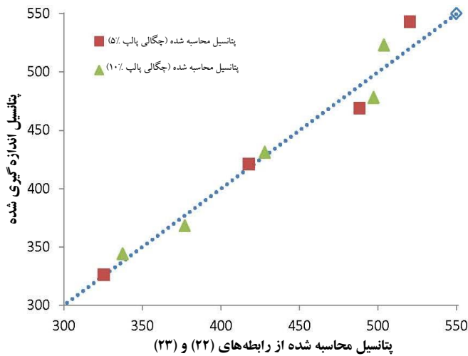
شکل ۴. مقایسه‌ی پتانسیل محاسبه شده به وسیله‌ی مدل پتانسیل ترکیبی با پتانسیل اندازه گیری شده.
