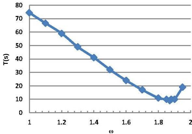
شکل ۲. رابطه بین زمان اجرای برنامه و \omega .
