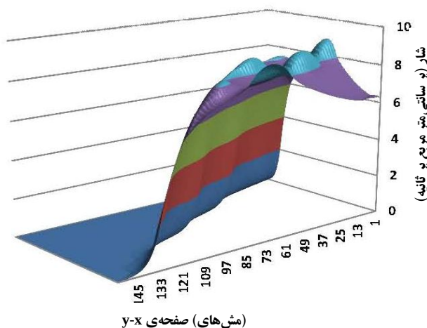
شکل ۷. توزیع شار نوترون‌های تند در مرکز قلب.
