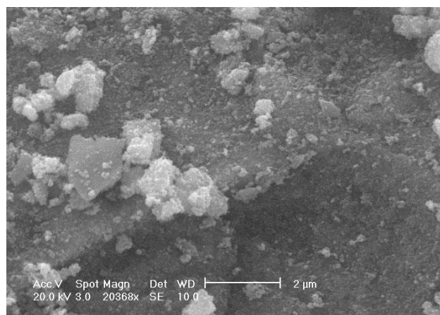
شکل ۲. ریزنگار الکترونی نانو ذرات ساخته شده (بزرگ‌نمایی ۲۰۰۰).
