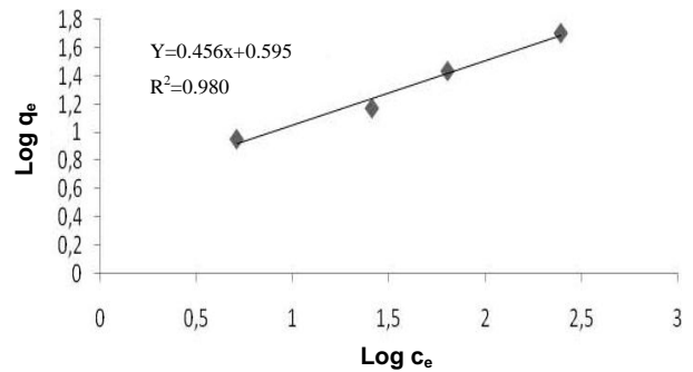
شکل ۱۰. ایزوترم فرندلیچ برای جذب توریم.
