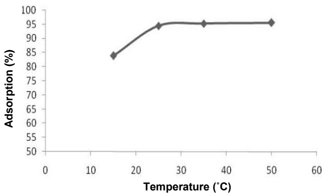
شکل ۱۳. اثر تغییر دما بر درصد جذب توریم.
