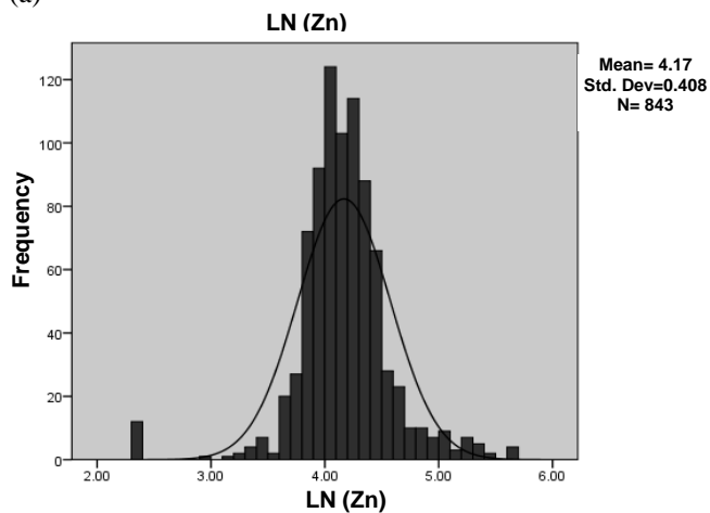
شکل ۲- هیستوگرام توزیع داده‌های خام (a) و بهنجار شده‌ی (b) عنصر روی.
