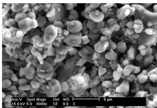
شکل ۸- عکس میکروسکوپ الکترونی نمونه شماره ۳، با بزرگ‌نمایی ۸۰۰۰.
