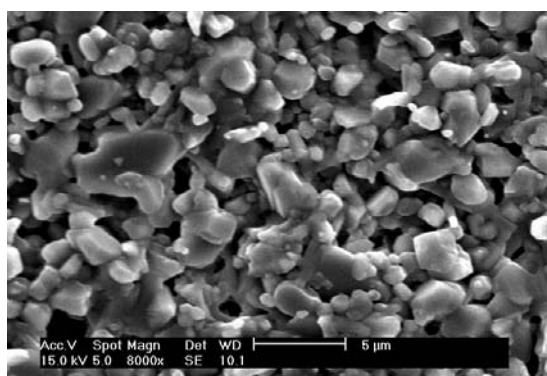
شکل ۷- عکس میکروسکوپ الکترونی نمونه شماره ۲، با بزرگ‌نمایی ۸۰۰۰.
