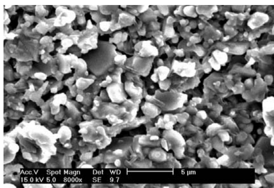
شکل ۶- عکس میکروسکوپ الکترونی نمونه شماره ۱، با بزرگ‌نمایی ۸۰۰۰.
