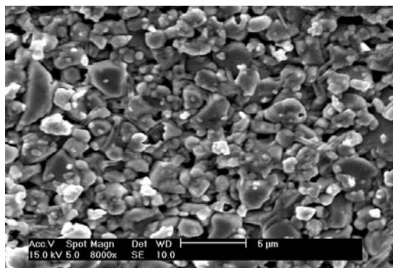
شکل ۹- عکس میکروسکوپ الکترونی نمونه شماره ۴، با بزرگ‌نمایی ۸۰۰۰.
