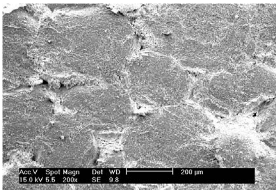
شکل ۲- عکس میکروسکوپ الکترونی نمونه شماره ۱، با بزرگنمایی ۲۰۰.
