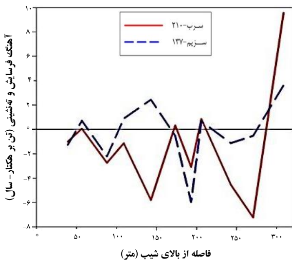
شکل ۵. آهنک فرسایش و ته‌نشینی برآورد شده (تن بر هکتار-سال) با استفاده از دو رادیونوکلید سزیم-۱۳۷ و سرب-۲۱۰ اضافی در امتداد سه ترانسکت.
