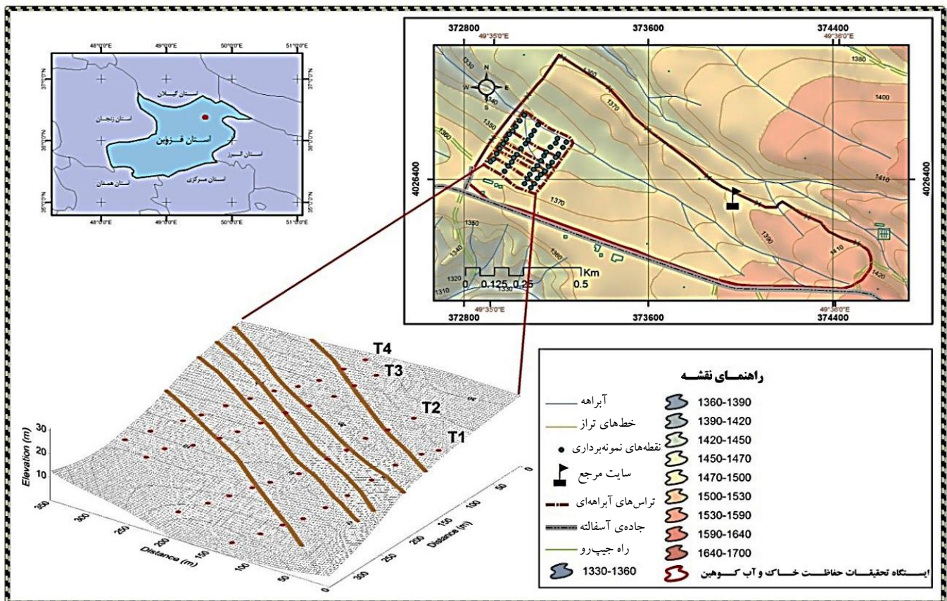
شکل ۱. موقعیت جغرافیایی ایستگاه تحقیقات حفاظت خاک و آب دانشگاه تهران، محل مرجع، تراس‌های آبراه‌ای و نقطه‌های نمونه‌برداری بر روی ترانسکت‌ها (T1 تا T4).
