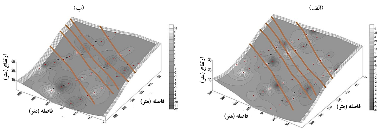
شکل ۴. نقشه‌ی آهنگ توزیع مجدد خاک (تن بر هکتار بر سال) برآورد شده به وسیله‌ی مدل موازنه‌ی جرم ۲ در روش‌های (الف) سزیم-۱۳۷ و (ب) سرب-۲۱۰ اضافی (مقدارهای منفی نشان‌دهنده‌ی فرسایش و مقدارهای مثبت نشان‌دهنده‌ی ته‌نشینی هستند).
