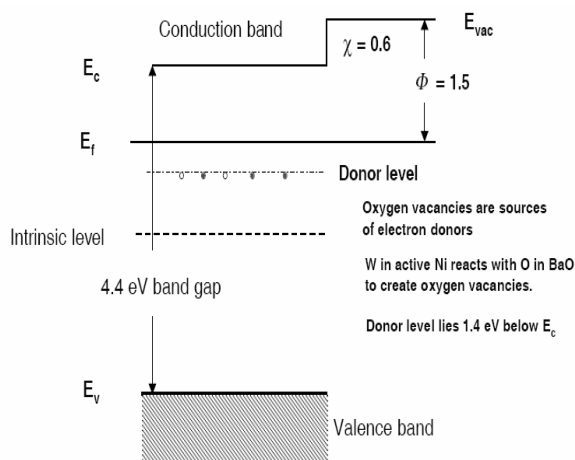
شکل ۱- مدل کاتد اکسیدی.
