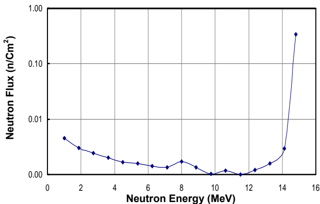
طیف انرژی نوترون پس از عبور از پوشش فولادی و آب و پوشش پلاستیکی.
