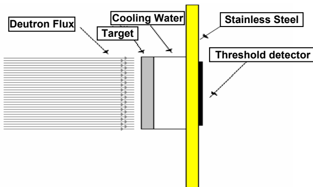
طرز قرار گرفتن هدف در مقابل شار دوترون.
