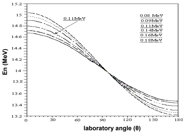
نمودار تغییرات انرژی نوترون برحسب زوایای مختلف برخورد دوترون به تریتیوم در انرژیهای مختلف دوترون.
