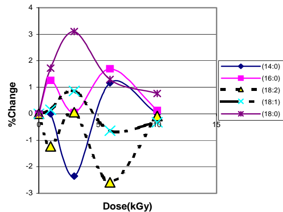
شکل ۳- درصد تغییرات اسیدهای چرب موجود در گوشت بر حسب دز.
