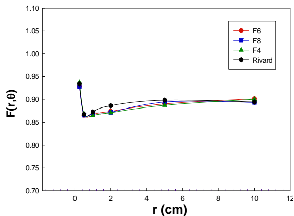
شکل ۵ - نمودار تابع ناهمسانگردی " F(r, \theta) " در زاویه ۳۰ درجه بر
