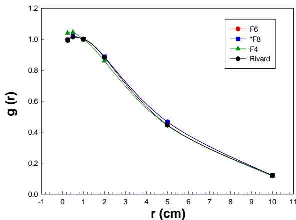
شکل ۳ - نمودار تابع دز شعاعی " g(r) " بر حسب فاصله و مقایسه آنها با
