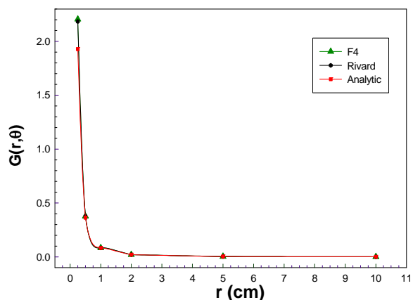
شکل ۴ - نمودار تابع آرایش هندسی " G(R, \theta) " در زاویه ۳۰ درجه بر حسب
