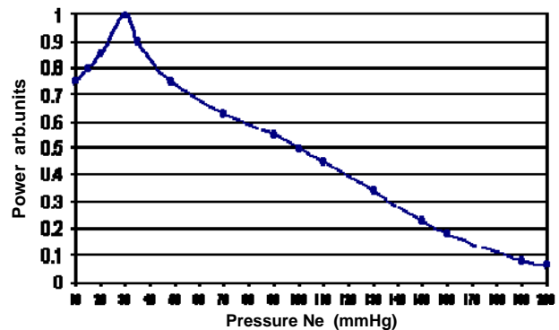
شکل ۳- وابستگی توان خروجی به فشار گاز نئون.
