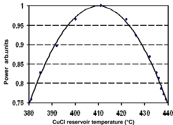
شکل ۴- توان خروجی بر حسب دمای مخزن نمک.
