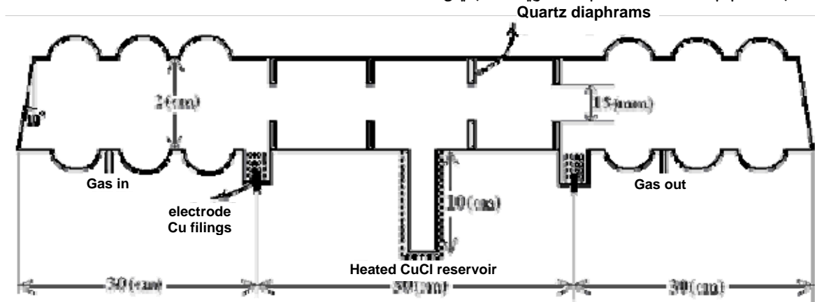
شکل ۱- طرحواره لیزر کلرید مس.
