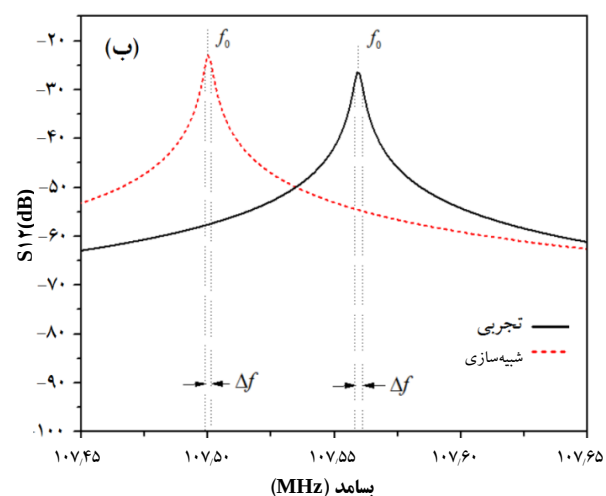
شکل ۱۳. (الف) بسامد تشدید اندازه‌گیری شده توسط پارامتر S_{11} پس از نصب کوپلر جفت‌ساز توان، (ب) اندازه‌گیری ضریب کیفیت براساس اندازه‌گیری پارامتر S_{12} در کاواک ساخته شده حاصل از نتایج تجربی و شبیه‌سازی با نرم‌افزار سی.اس.تی.
