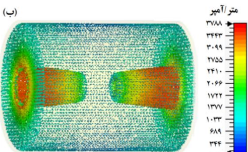
شکل ۱۲. (الف) شکل سه‌بعدی میدان الکتریکی برحسب ولت بر متر و (ب) جریان سطحی برحسب آمپر بر متر، در کاواک شبیه‌سازی شده با استفاده از نرم‌افزار سی.اس.تی.
