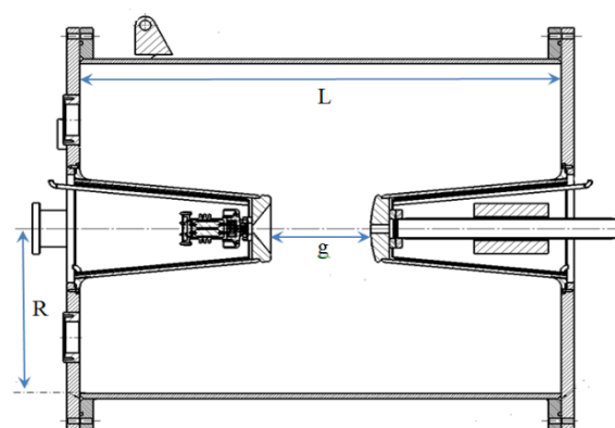
شکل ۲. برشی از طرح ابعادی کاواک طراحی شده.
