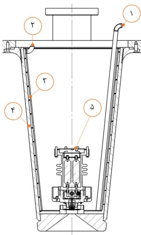
شکل ۴. نمایی از نحوه‌ی خنک‌سازی دماغه‌ی کاواک طراحی شده و مؤلفه‌های آن شامل: (۱) ورودی آب خنک‌کننده، (۲) خروجی آب خنک‌کننده، (۳) جداره‌ی مسیر چرخش آب در امتداد دماغه، (۴) دیواره‌ی دماغه در داخل کاواک، (۵) تفنگ الکترونی.
