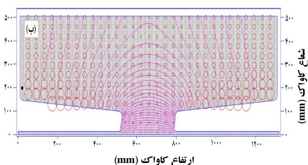
شکل ۱۱. (الف) شکل دوبعدی میدان الکتریکی و (ب) میدان مغناطیسی، در کاواک شبیه‌سازی شده با استفاده از نرم‌افزار سوپرفیش.
