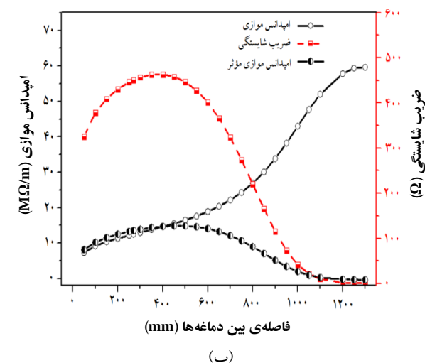
شکل ۸. الف) تأثیر فاصله‌ی دماغه‌ها بر بسامد و ضریب زمان عبور، (ب) امپدانس موازی، امپدانس موازی مؤثر و ضریب شایستگی (R/Q).
