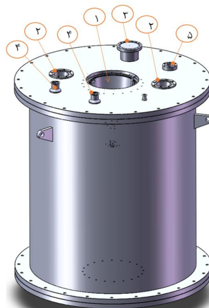
شکل ۳. (۱) طرح سه‌بعدی کاواک طراحی شده که در آن دماغه‌ی اتصال تفنگ الکترونی نشان داده شده است، (۲) محل اتصال کوپلرهای جفت شده‌ی توان، (۳) محل اتصال پمپ خلأ، (۴) محل اتصال سنسورهای خلأ، (۵) محل اتصال فیدبک RF.
