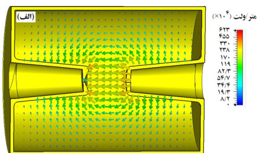
شکل ۱۱. (الف) شکل دوبعدی میدان الکتریکی و (ب) میدان مغناطیسی، در کاواک شبیه‌سازی شده با استفاده از نرم‌افزار سوپرفیش.
