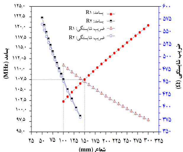
شکل ۶. تأثیر مخروطی کردن دماغه بر بسامد و ضریب شایستگی کاواک (R/Q).
