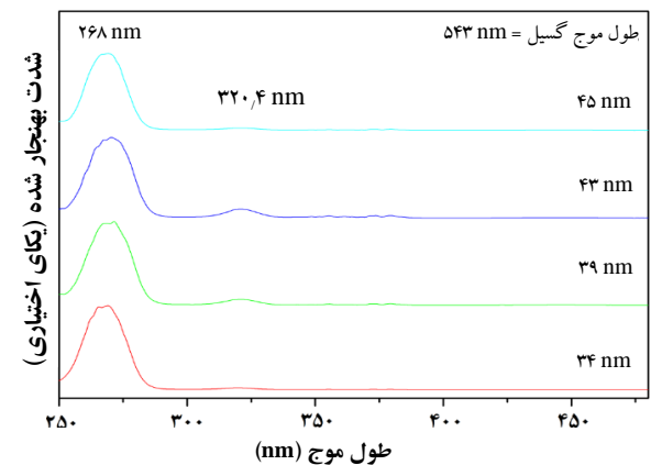
شکل ۶. طیف برانگیختگی بهنجار شده‌ی نانوبلورهای مختلف لوتسیم آلومینیم گارنت آلائیده شده با تربیم برای طول موج گسیل ۵۴۳ nm.
