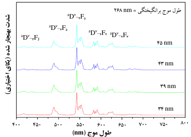
شکل ۵. طیف نشری بهنجار شده‌ی نانوبلورهای مختلف لوتسیم آلومینیم گارنت آلائیده شده با تربیم برای طول موج برانگیختگی ۲۶۸ nm.
