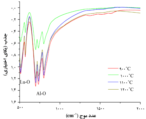
شکل ۳. طیف تبدیل فوریه ی زیرقرمز (FTIR) نانوبلورهای گارنت آلائیده شده با تربیم، تهیه شده در دماهای مختلف به روش هم رسوبی.
