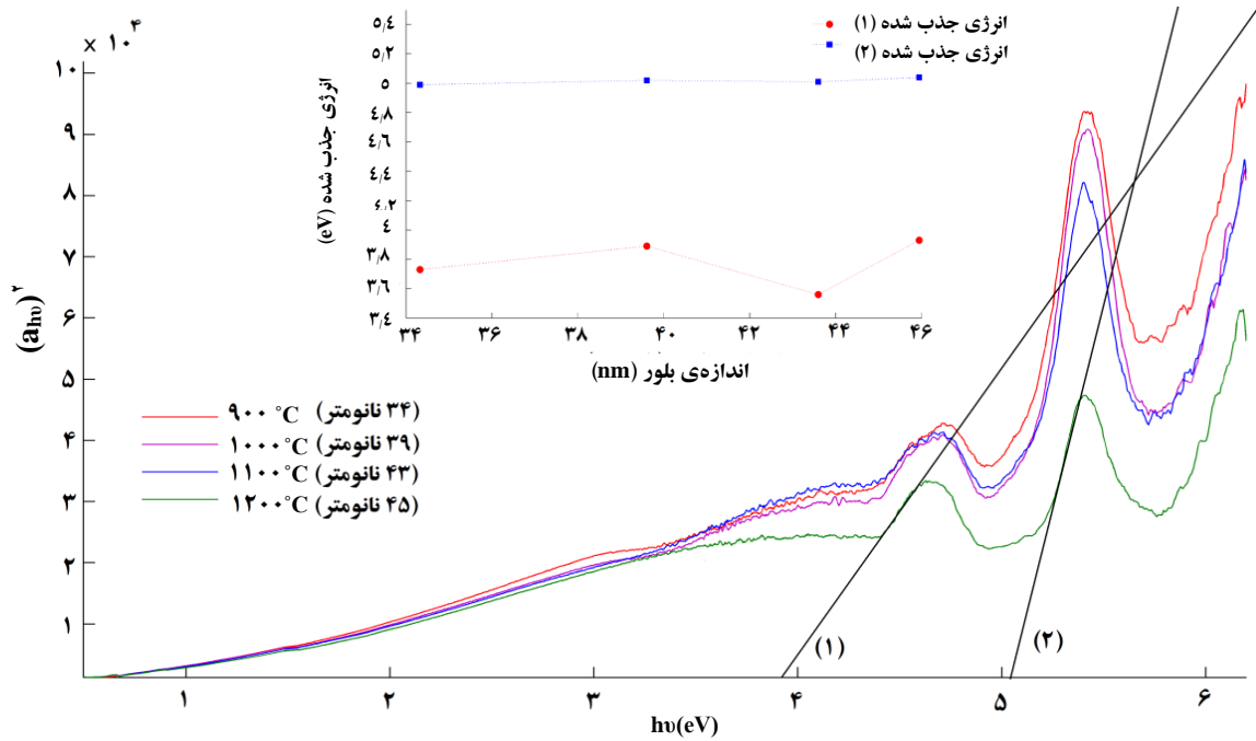
شکل ۴. طیف دیدگانی- فرابنفش و مقادیرهای انرژی جذب شده به دست آمده از نانوبلورهای مختلف لوتسیم آلومینیم گارنت آلائیده شده با تربیم.
