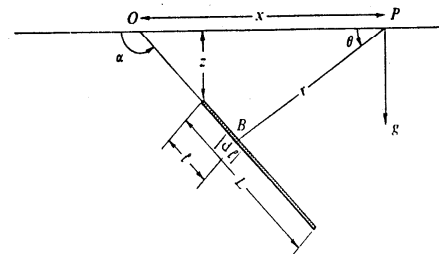
شکل ۲- شکل مربوط به میله نازک
