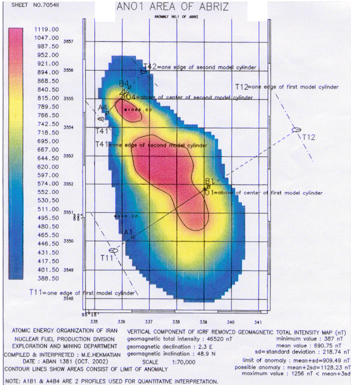
شکل ۵ - نقشه مؤلفه عمودی شدت میدان مغناطیسی زمین نابهنجاری ۱ ناحیه آبریز که تصحیح IGRF روی آن اعمال شده است
