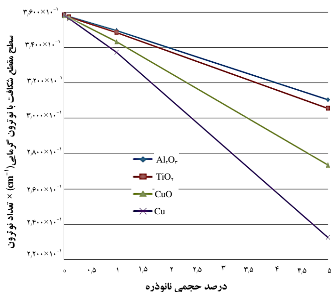
شکل ۷. رابطه‌ی بین سطح مقطع ماکروسکوپی شکافت با نوترون‌های گرمایی ضرب در تعداد متوسط نوترون‌های گرمایی حاصل از شکافت ( \Sigma_f ) در یک میله سوخت و درصد حجمی نانوذره.
