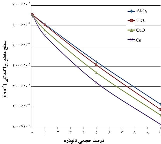
شکل ۳. رابطه‌ی بین سطح مقطع پراکندگی ماکروسکوپی نوترون‌های گرمایی در کانال کندساز و درصد حجمی نانوذره.
