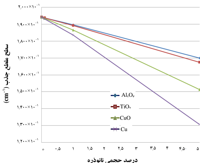
شکل ۵. رابطه‌ی بین ضریب پخش نوترون‌های گرمایی در کانال کندساز و درصد حجمی نانوذره.
