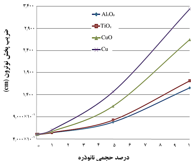
شکل ۶. رابطه‌ی بین سطح مقطع ماکروسکوپی جذب نوترون‌های گرمایی در یک میله سوخت و درصد حجمی نانوذره.
