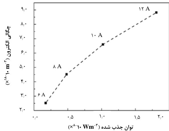
شکل ۱۰. تغییرات چگالی پلاسما و توان جذب شده با جریان اعمال شده به آنتن.
