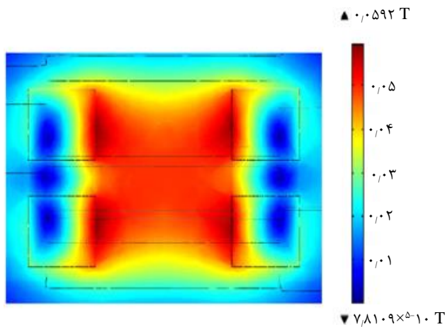
شکل ۲. میدان مغناطیسی یکنواخت شبیه‌سازی شده در بین پیچه‌های مغناطیسی بر روی خط مرکز پیچه‌ها.
