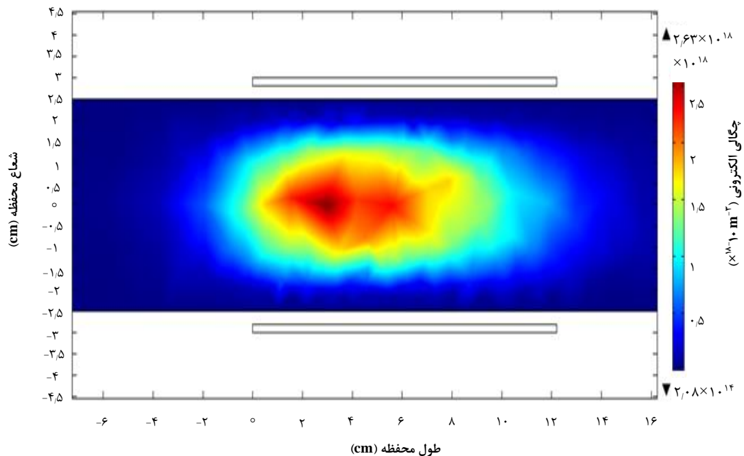
شکل ۵. سیستم پلاسمای هلیکون شبیه‌سازی شده با آنتن ناگویا با چگالی 2.63 \times 10^{18} \text{ m}^{-3} ، میدان مغناطیسی ثابت 600 \text{ G} ، بسامد 13.56 \text{ MHz} و توان 1.5 \text{ kW} .
