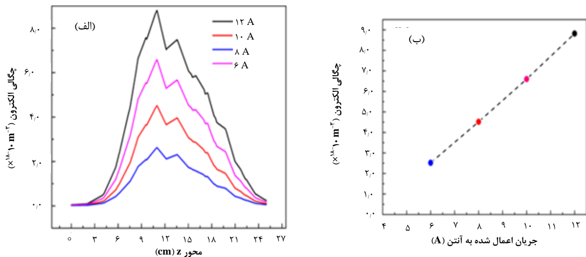
شکل ۹. (الف): توزیع محوری چگالی پلازما برای جریان‌های مختلف ۶A (آبی)، ۸A (قرمز)، ۱۰A (صورتی)، و ۱۲A (سیاه) و (ب): رابطه‌ی بین بیشینه‌ی چگالی پلازما و جریان اعمال شده به آنتن ناگویا (ب).
