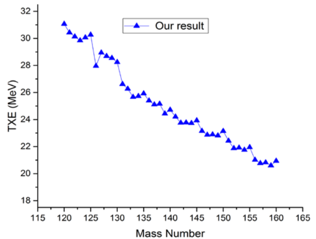
شکل ۴. انرژی تحریکی کل محاسبه شده برای شکافت نوترونی اورانیم-۲۳۸.
