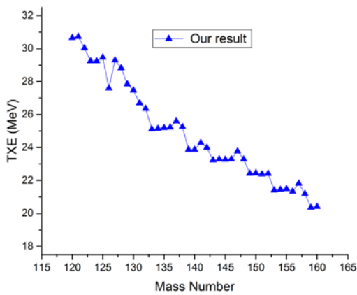
شکل ۶. انرژی تحریکی کل محاسبه شده برای شکافت نوترونی اورانیم-۲۳۸.
