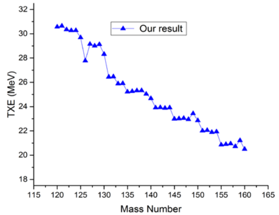
شکل ۳. انرژی تحریکی کل محاسبه شده برای شکافت نوترونی اورانیم-۲۳۸.
